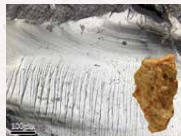
砂原遺跡（島根県）出土の剥片と顕微鏡で観察した斑晶
