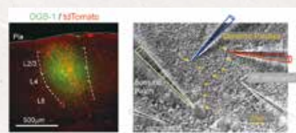
大脳皮質のクローン細胞群（橙色、左図）と小脳神経細胞からの多重同時パッチクランプ記録（右図） Clonally-related neurons in the cerebral cortex (orange, left) & simultaneous multiple patch-clamp recordings from a single cerebellar Purkinje cell (right).
