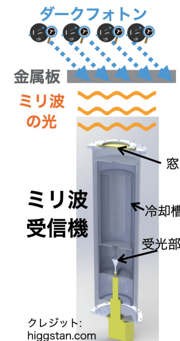
図1 ダークフォトンの検出方法。金属板でダークフォトンが微弱なミリ波の光に転換される。開発する高感度ミリ波受信機で、この光を捉える。
